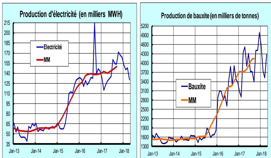
GRAPHIQUE 2.1 : ÉVOLUTION DES PRODUCTIONS DE BAUXITE & D'ÉLECTRICITÉ
